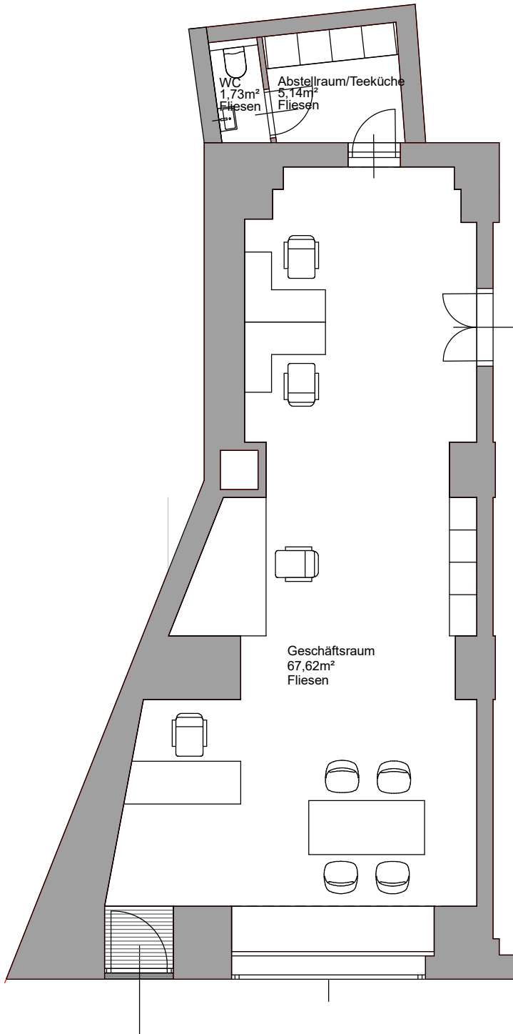
GRUNDRISS ERDGESCHOSS
