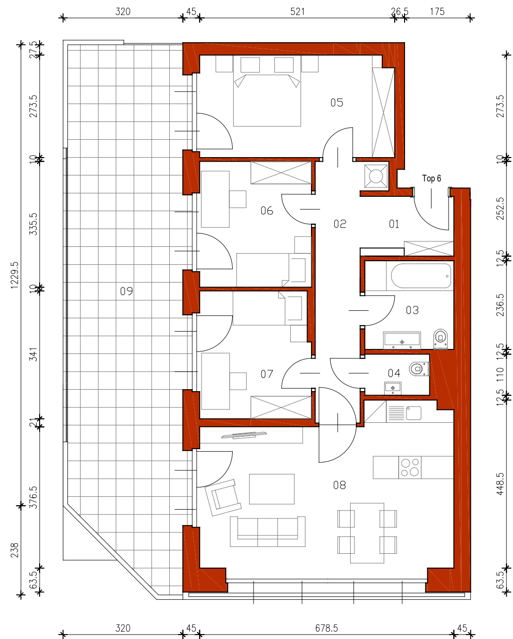
GRUNDRISS 1.DACHGESCHOSS
